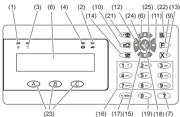
Figuur 2: ATS1135-gebruikersinterface
